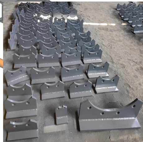
(d) Valve Holders
